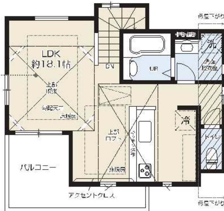
2F / 40.78m 2 (約12.33坪)
